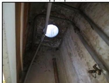
Photo N° 97 AMIANTE CIMENT -- PALIER 7 Conduits de ventilation Ventilation haute (Fibres-ciment)
